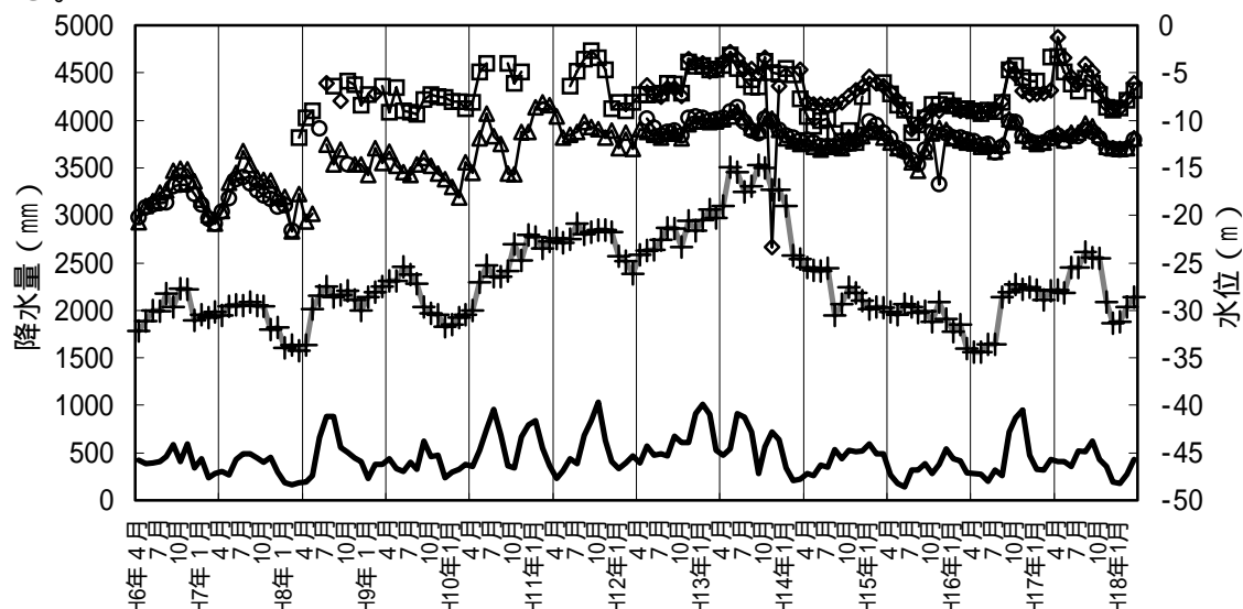
図4-13 福里流域の水源井戸の水位変動
