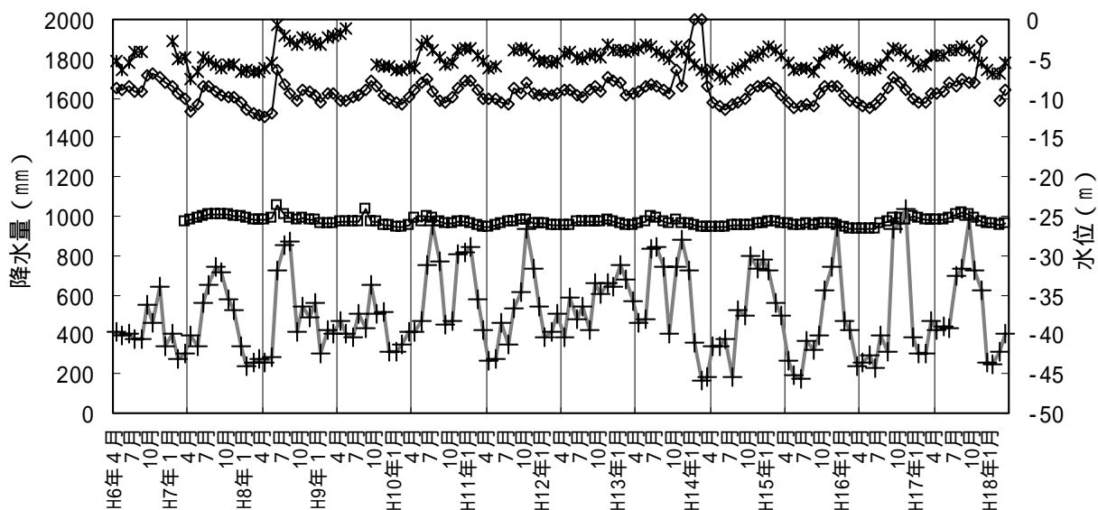
図4-12 白川田流域の水源井戸の水位変動
