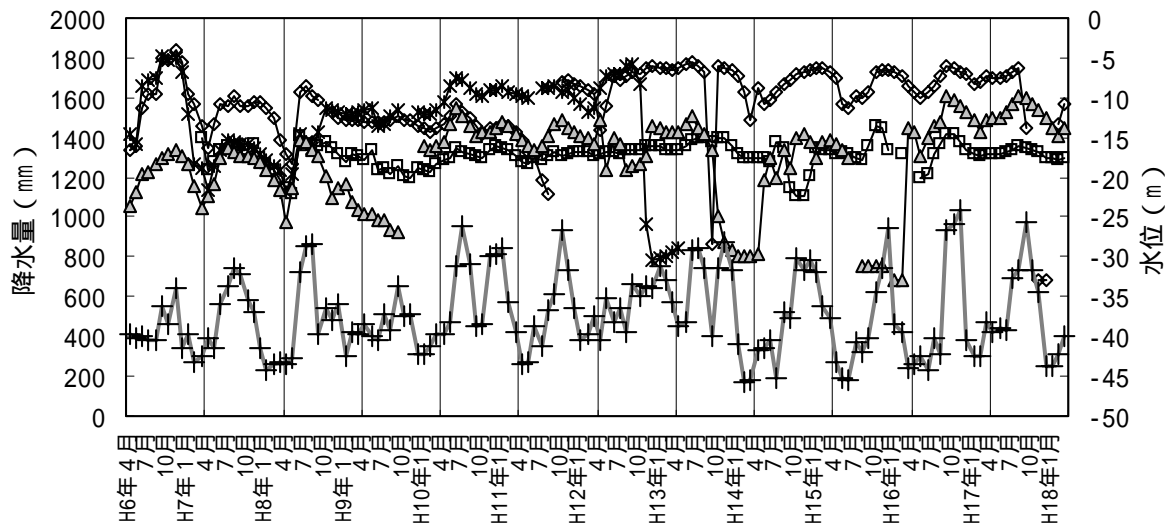
図4-11 東添道流域の水源井戸の水位変動
