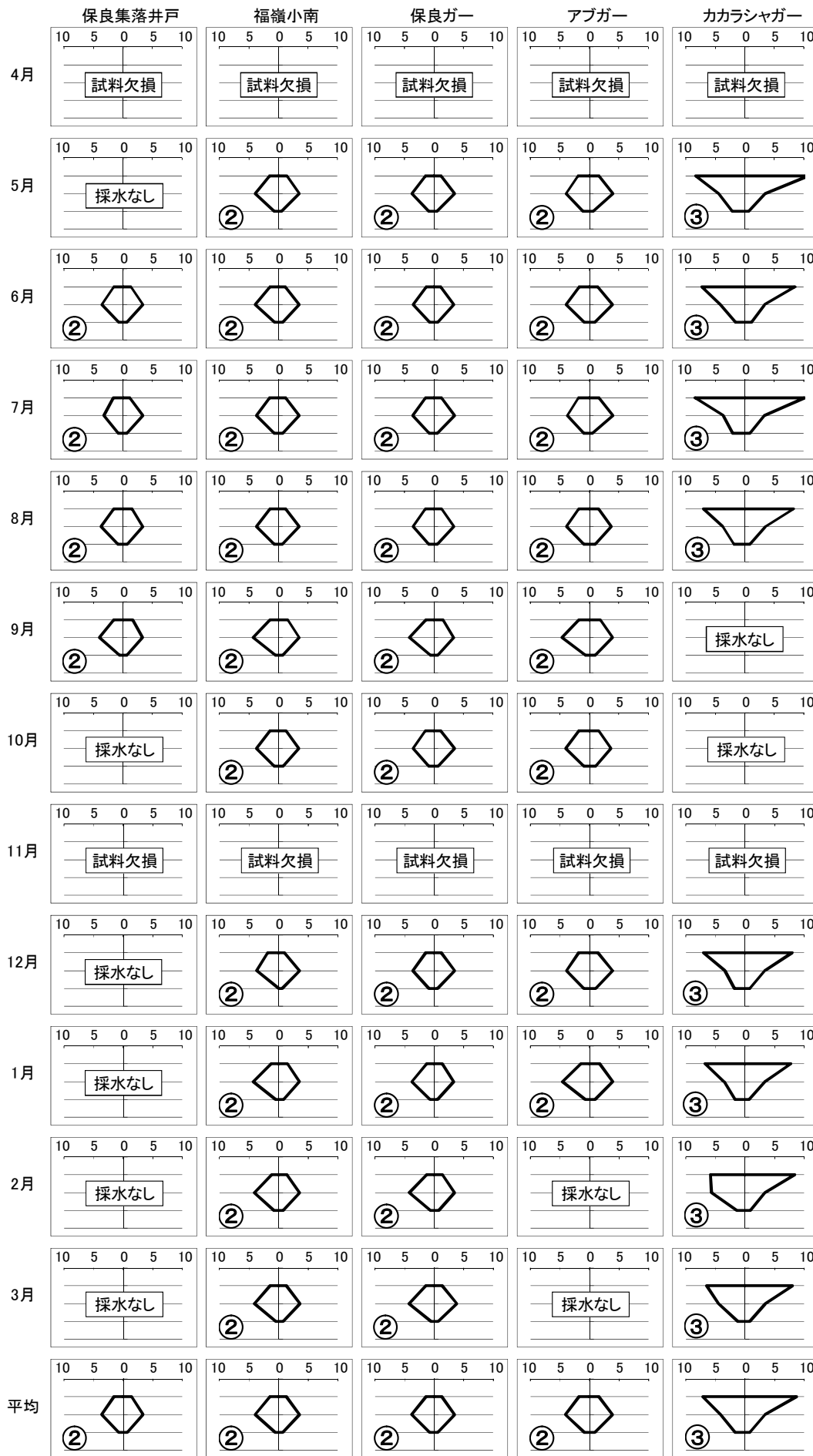
図4-4-9 各地点のイオンバランス(ヘキサダイアグラム)
